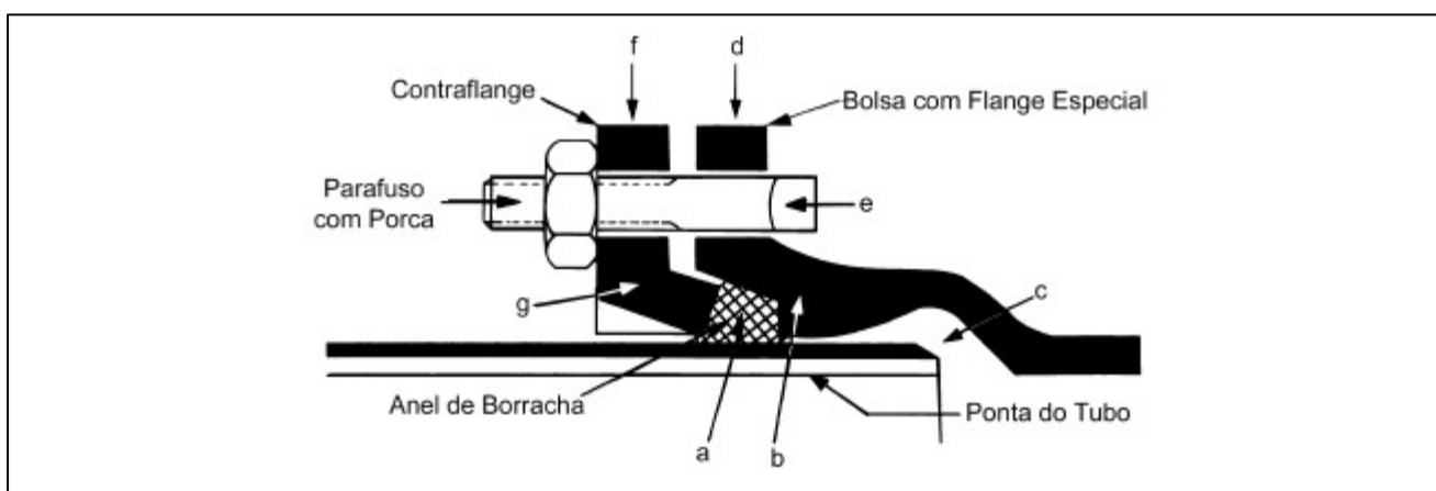
Fig. 11 - Junta Mecânica.
