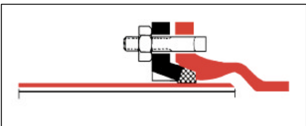
Fig. 03. Junta Mecânica
