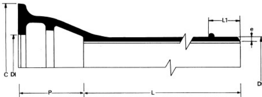
Tubos de Ferro Fundido Dúctil, Classe K-9 com Junta Elástica Travada
