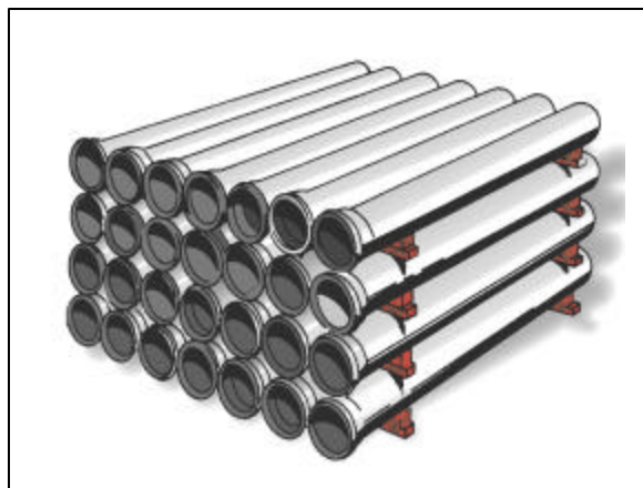
Fig. 04. Armazenagem em leitos superpostos, com bolsas no mesmo sentido.
