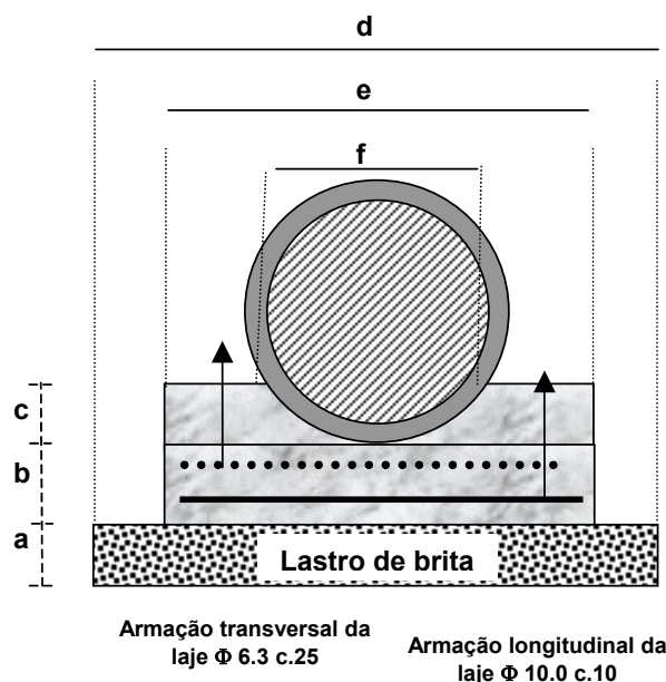
Figura 02. Lastró, laje e berço de concreto - dimensões em função do diâmetro do tubo
