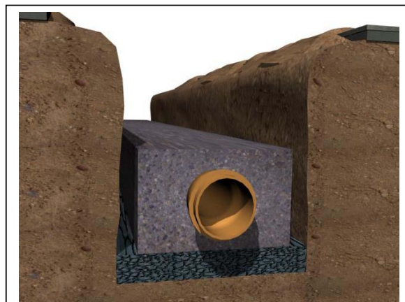
ENVELOPE DE CONCRETO
